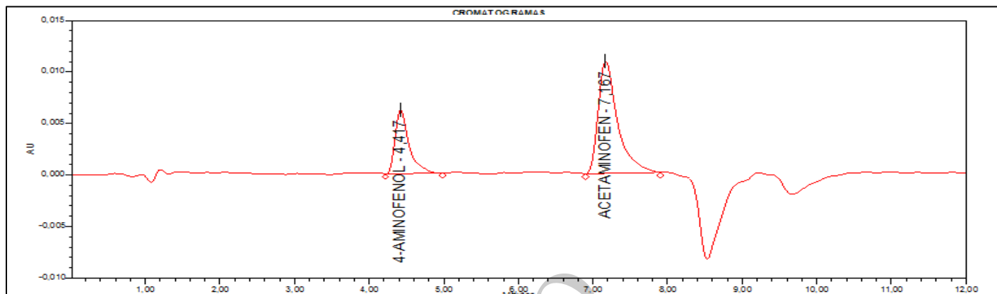
Figura 3. Cromatograma típico de la solución estándar para 4- Aminofenol
